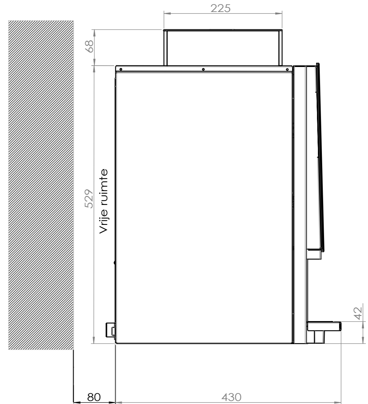
Zijaanzicht
